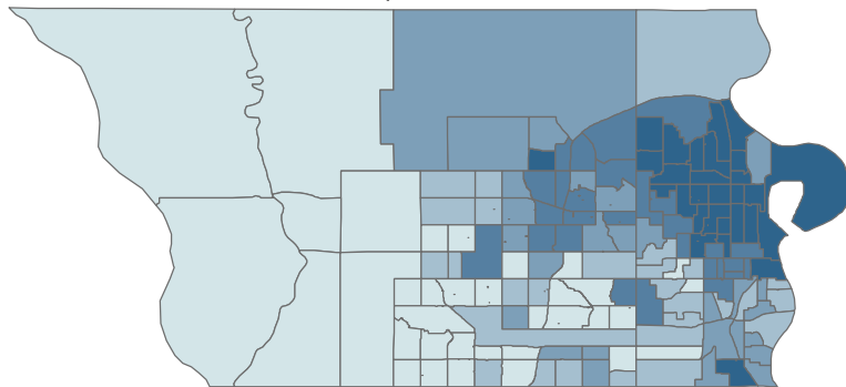
Quantile
